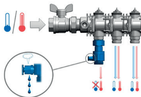
Schema debiet vs. temperatuur
