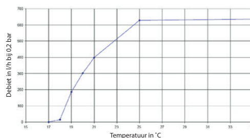
Schema debiet vs. temperatuur
