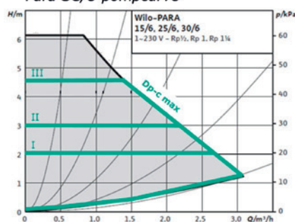
Para SC/U pompcurve
