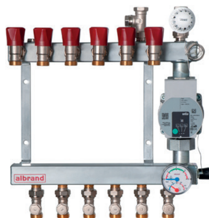
Voorbeeld van verdeler met pomp i.c.m. CV ketel
