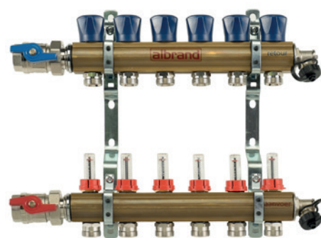
Voorbeeld van verdeler zonder pomp i.c.m. warmtepomp
